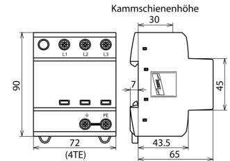
Maßbild DSH TNC 255
