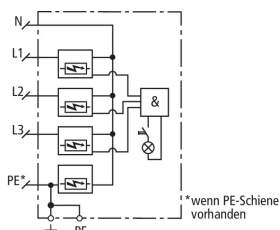
Prinzipschaltbild DSH ZP TT 255
