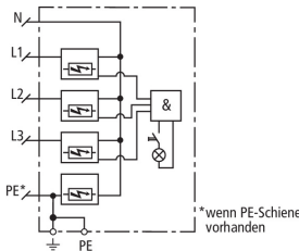
Prinzipialschaltbild DSH ZP B TT 255
