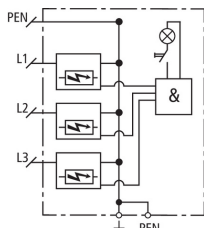
Prinzipschaltbild DSH ZP B TNC 255
