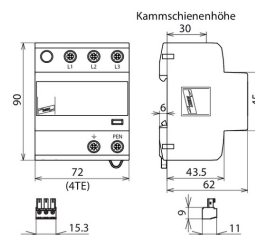
Maßbild DSH B TNC 255 FM
