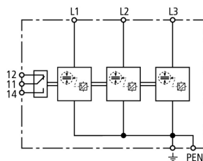
Prinzipschaltbild DSH B TNC 255 FM
